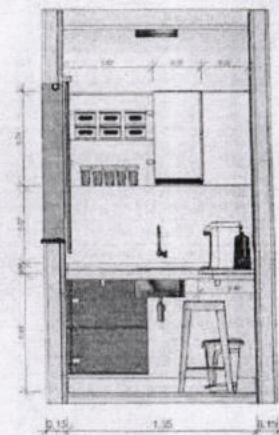
3 CORTE BB 1 : 35
