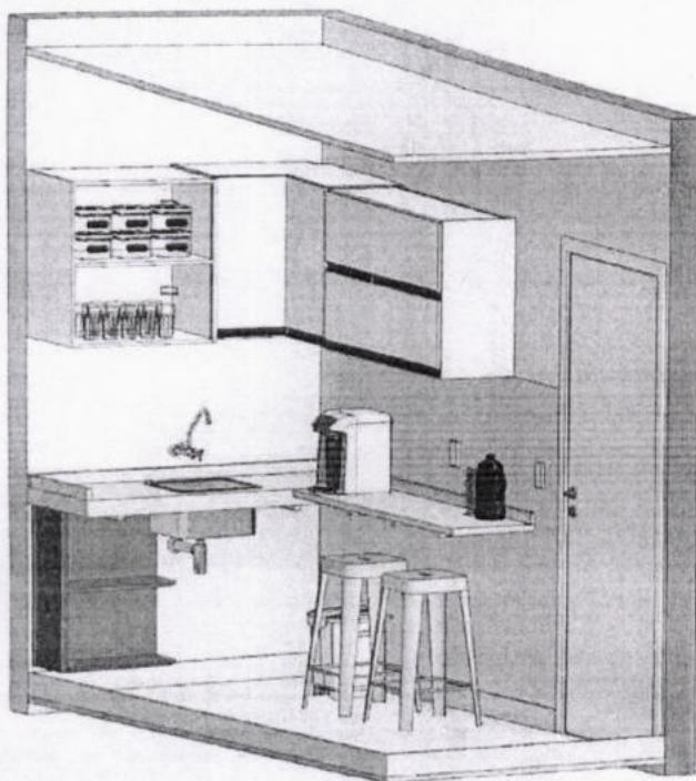
1 ISOMÉTRICA I
