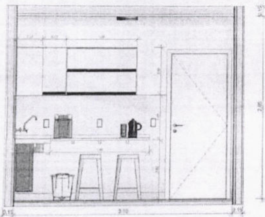
2 CORTE AA 1 : 35
